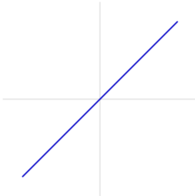
Gambar 1: Grafik fungsi linear
