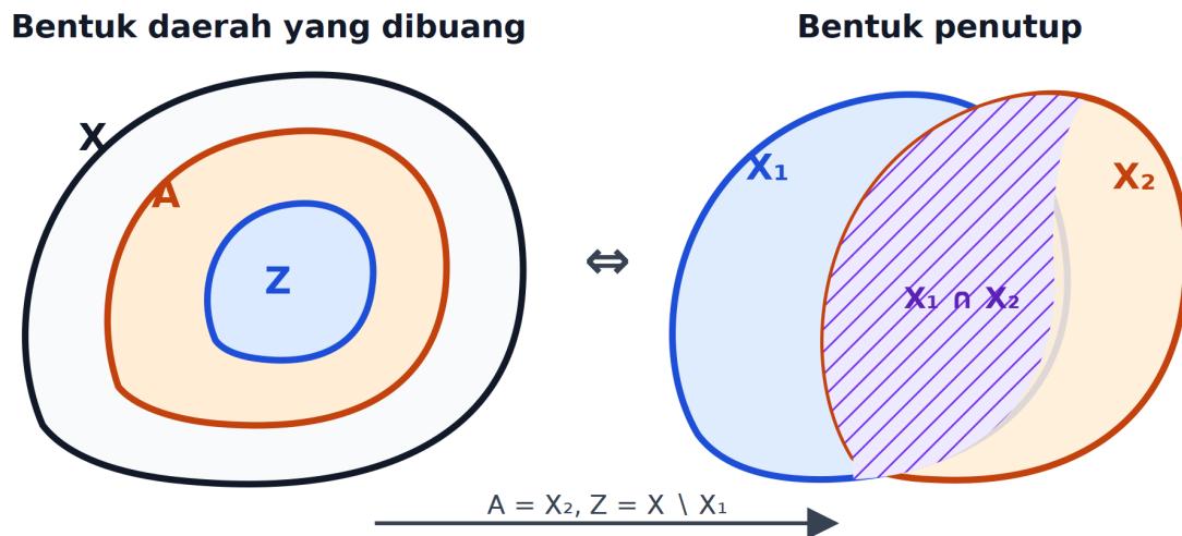
Gambar 7: Gambar ulang aksesibel dua rumusan eksisi: daerah Z di dalam A di dalam X , dan penutup X satu- X dua dengan daerah irisan.
