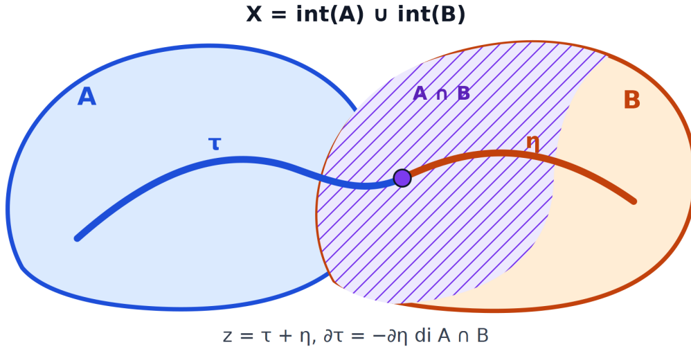
Gambar 8: Gambar ulang aksesibel penutup Mayer–Vietoris: A dan B menutupi X ; rantai z dipotong menjadi \tau di A dan \eta di B dengan batas berlawanan pada irisan.
