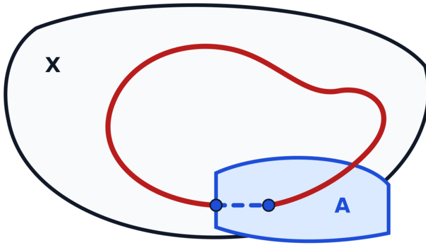
Gambar 5: Redraw aksesibel batas relatif: batas merah ditutup oleh ruas biru putus-putus yang terletak di A.
