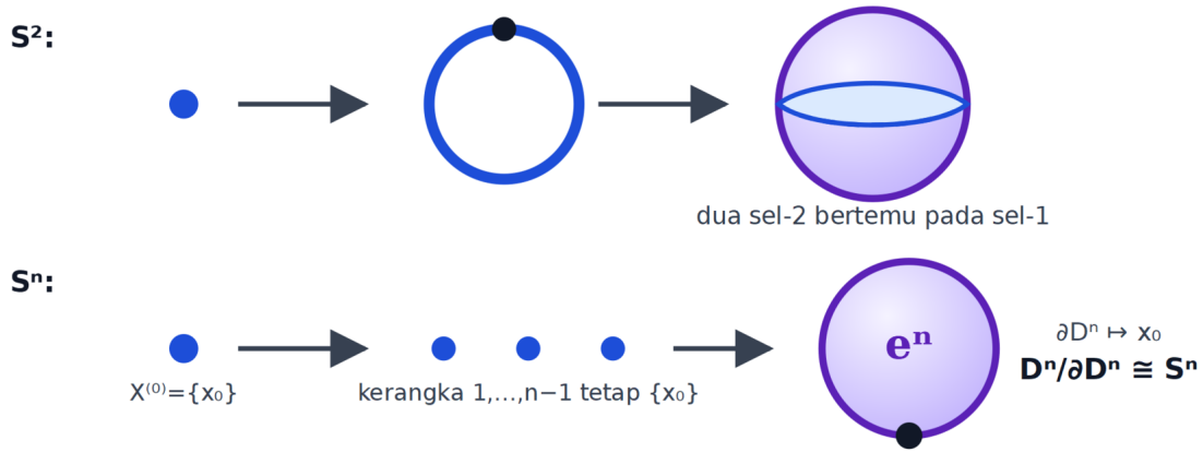
Gambar 14: Gambar ulang aksesibel dua struktur CW pada sfera: struktur empat-sel pada S dua dan struktur minimal dua-sel pada S^n .
