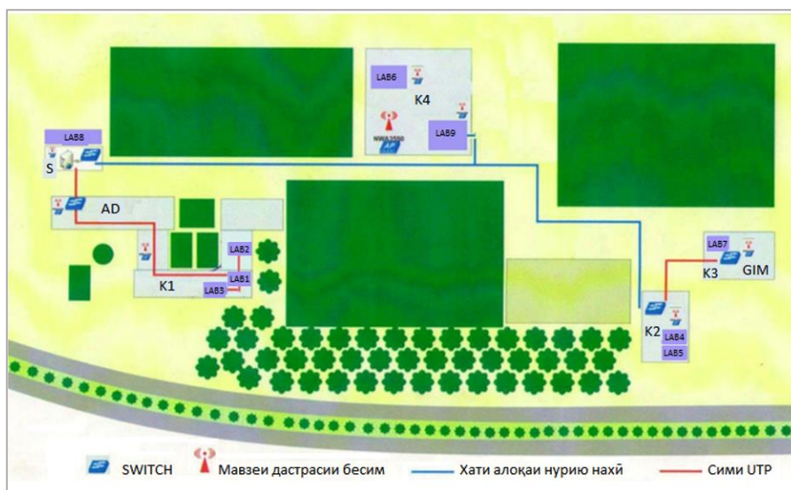
Расми 1. Нақшаи инфрасохтори иттилоотии шабакаи компютерии маҳаллии ДССХ.
