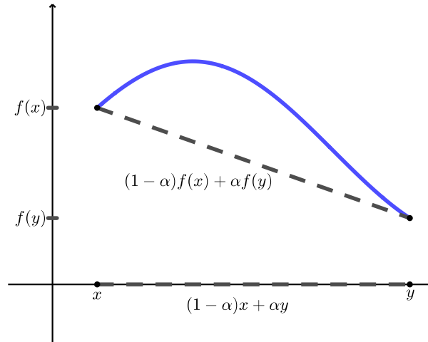
Gambar 3.12 Suatu fungsi cekung.
