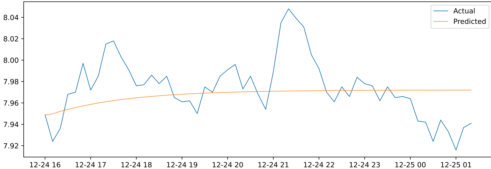
arima Actual vs Predicted pH
