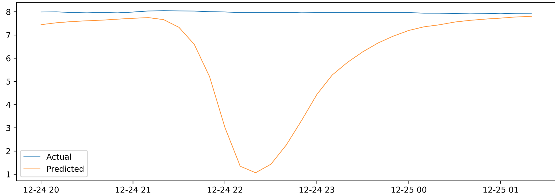
gru Actual vs Predicted pH
