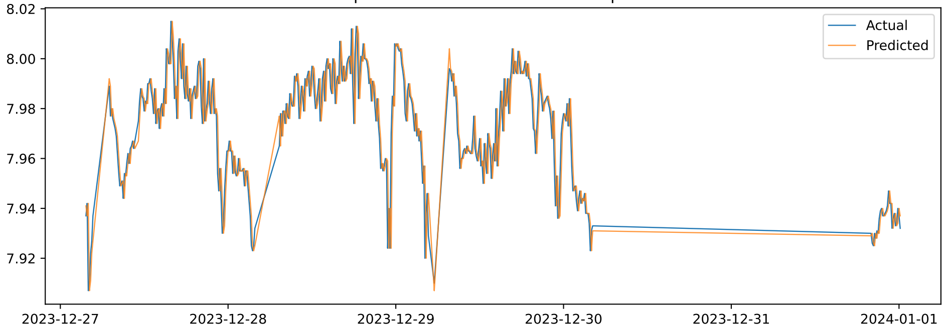
persistence Actual vs Predicted pH
