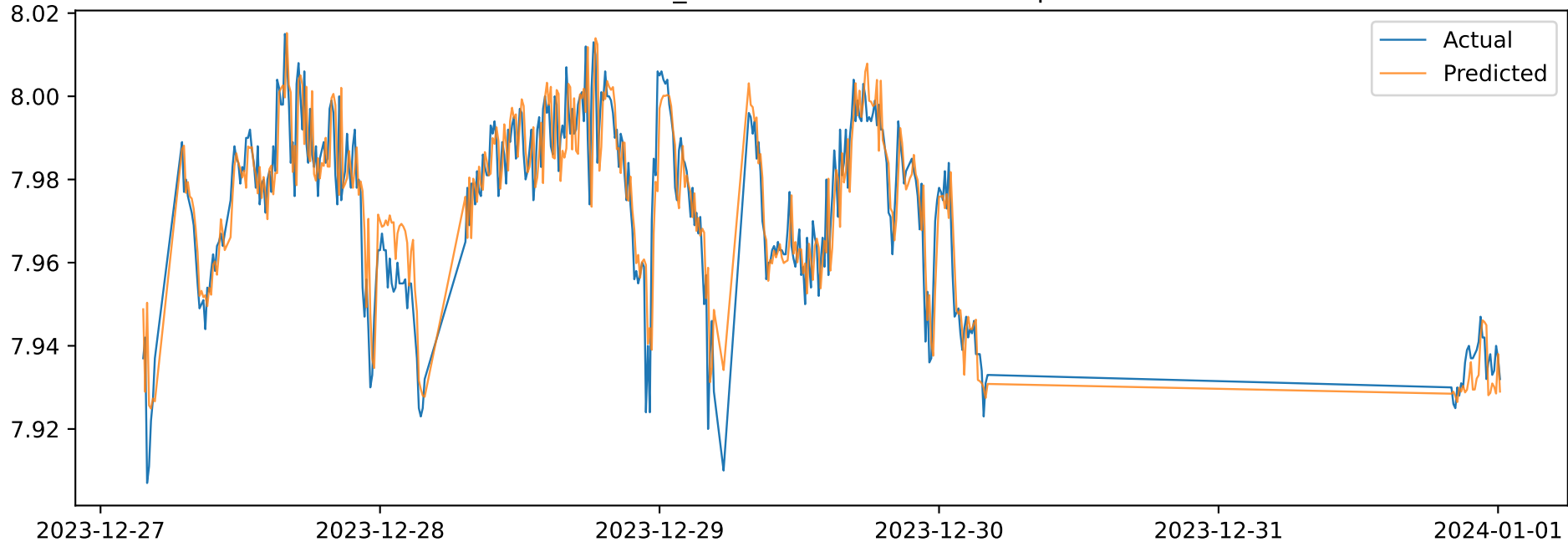
random_forest Actual vs Predicted pH
