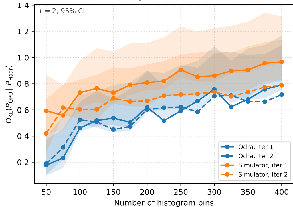
QPU vs Haar
