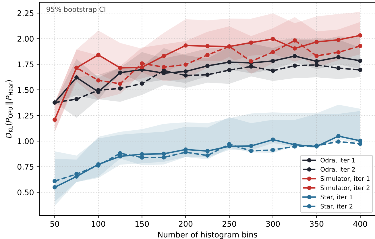
KL vs bins — depth L = 4 ( N = 60 , S = 2048 )
