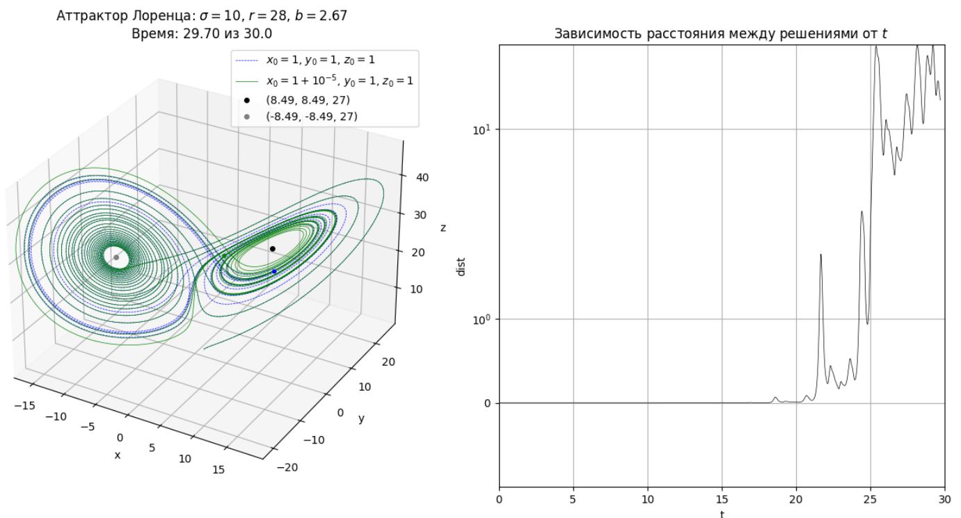
Рис. 1: Аттрактор Лоренца
