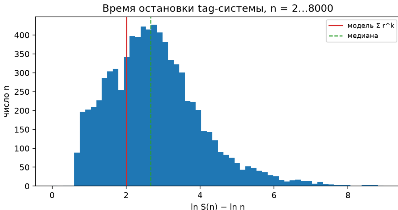
Рис. 3: \ln S(n) - \ln n для n \leq 8000
