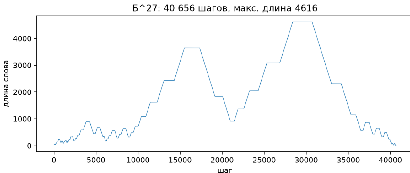
Рис. 4: Длина слова на траектории Б 27
