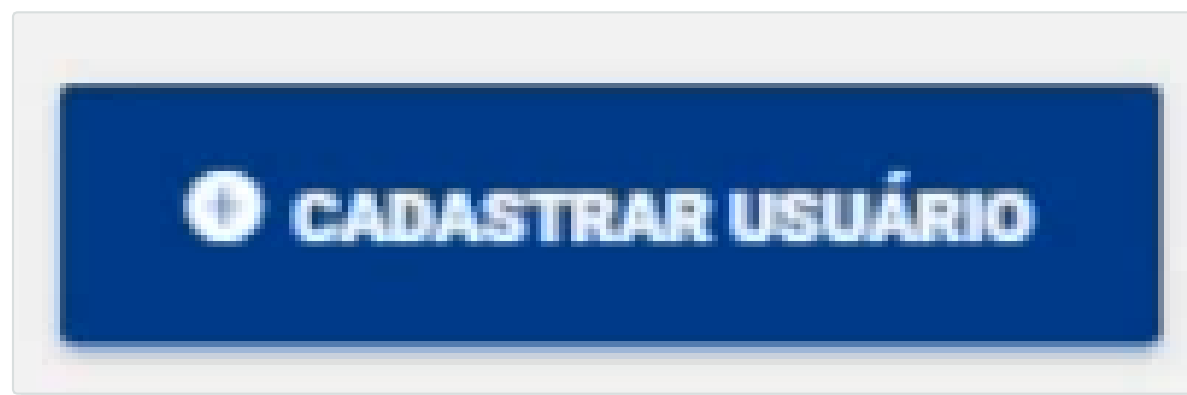
Cadastrar usuário
