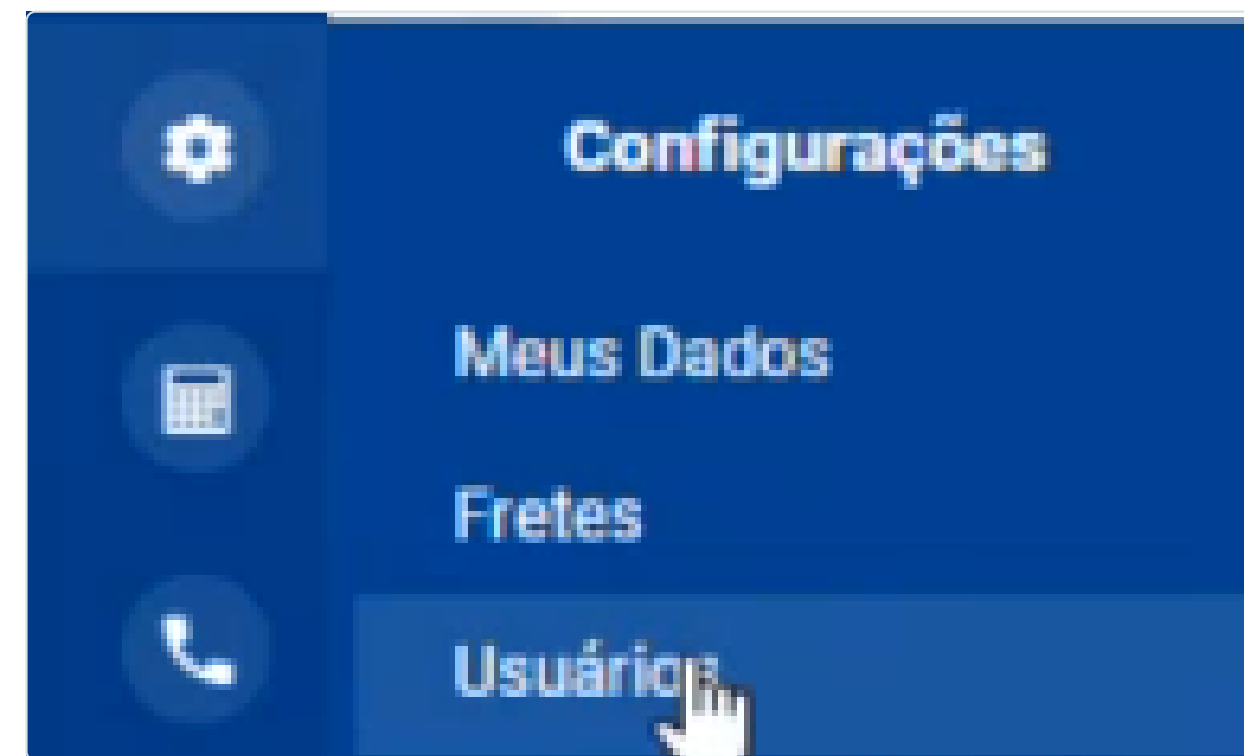
Configurações → Usuários
