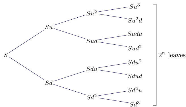
Figure 8.10.: Bushy tree : 追蹤的是 path 而不是股價。像 Su^2d 、 Sudu 、 Sdu^2 這些相同的股價，會以不同的 nodes 出現。
