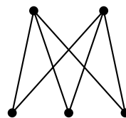
K_{2,3} : 6 edges
