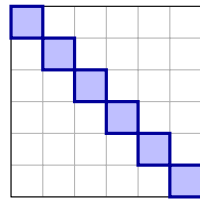
sizes (1, 1, 1, 1, 1, 1) per = 1
