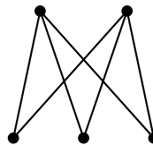
K_{2,3} : 6 edges
