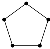
C_5 : 5 edges
