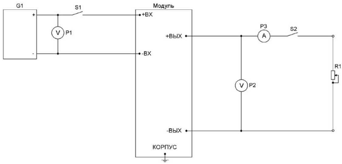
Схема измерения падения напряжения на модуле
