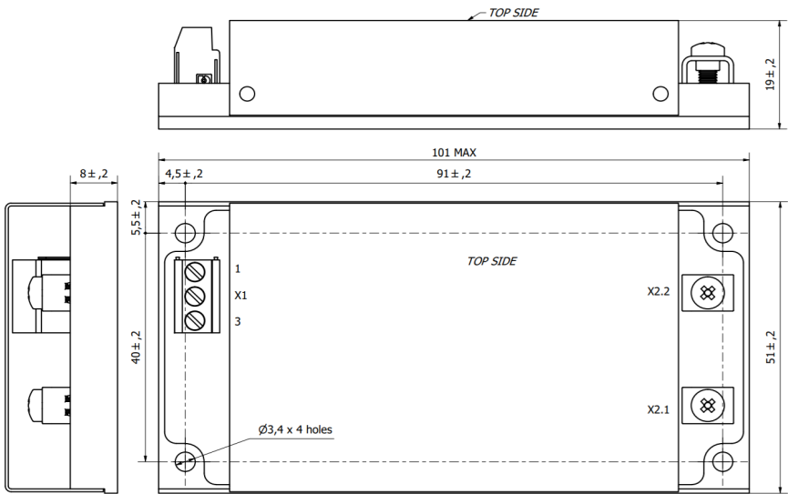
Рисунок В.1 - Габаритные, присоединительные и установочные размеры модулей JETAs30, JETAs40, JETAs60, одноканальное исполнение (индекс S), с клеммными колодками (индекс C)
