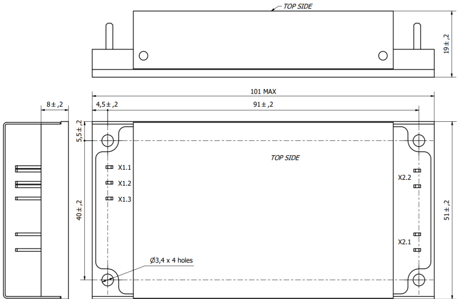
Рисунок В.4 - Габаритные, присоединительные и установочные размеры модулей JETAs30, JETAs40, JETAs60, одноканальное исполнение (индекс S), с ножевыми контактами (индекс Н)
