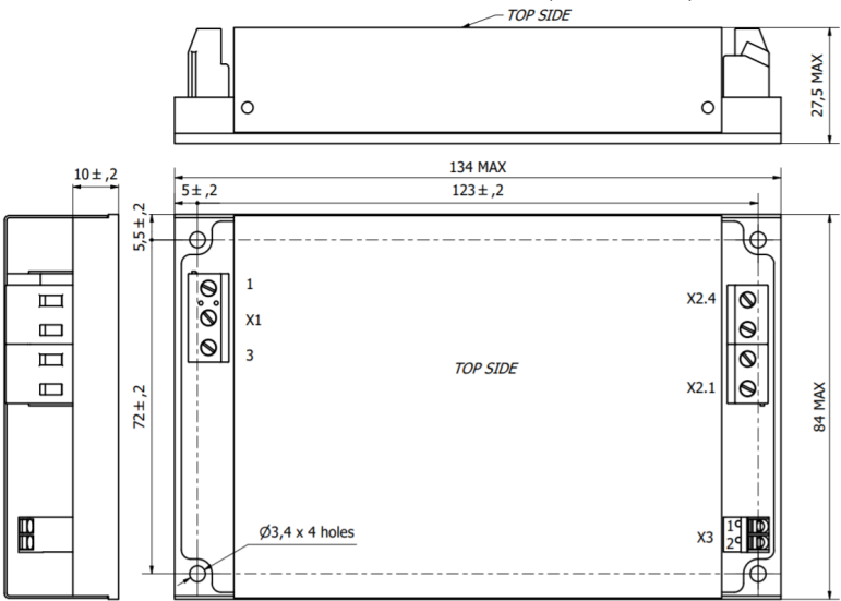
Рисунок Д.2 - Габаритные, присоединительные и установочные размеры модулей JETAs150, JETAs250, JETAs300, двухканальное исполнение (индекс D), с клеммными колодками (индекс C)
