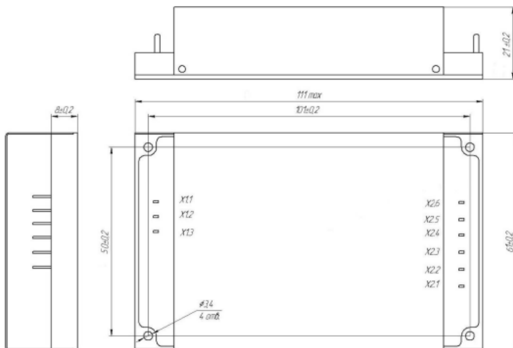
Рисунок Г.5 - Габаритные, присоединительные и установочные размеры модулей JETAs80, JETAs100, JETAs120, двухканальное исполнение (индекс D), с ножевыми контактами (индекс Н)
