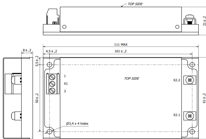
Рисунок Г.1 - Габаритные, присоединительные и установочные размеры модулей JETAs80, JETAs100, JETAs120, одноканальное исполнение (индекс S), с клеммными колодками (индекс C)
