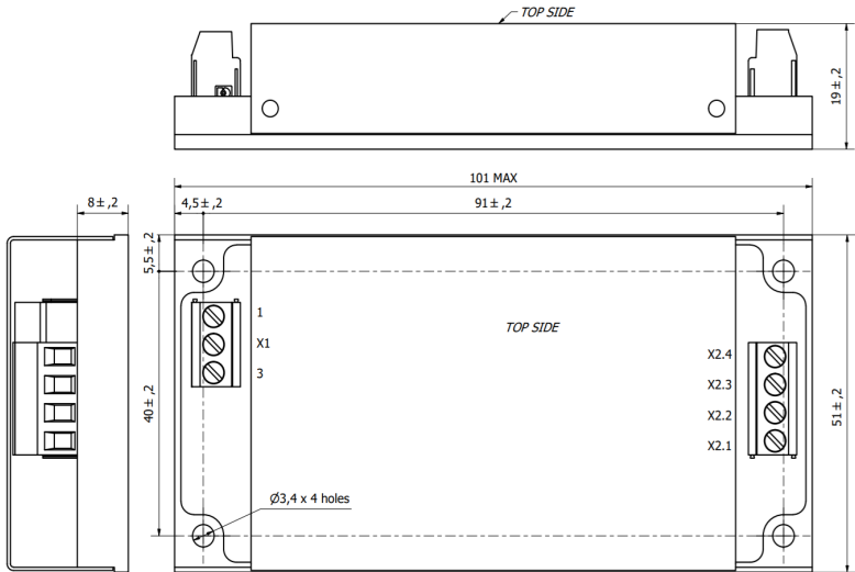
Рисунок В.2 - Габаритные, присоединительные и установочные размеры модулей JETAs30, JETAs40, JETAs60, двухканальное исполнение (индекс D), с клеммными колодками (индекс C)
