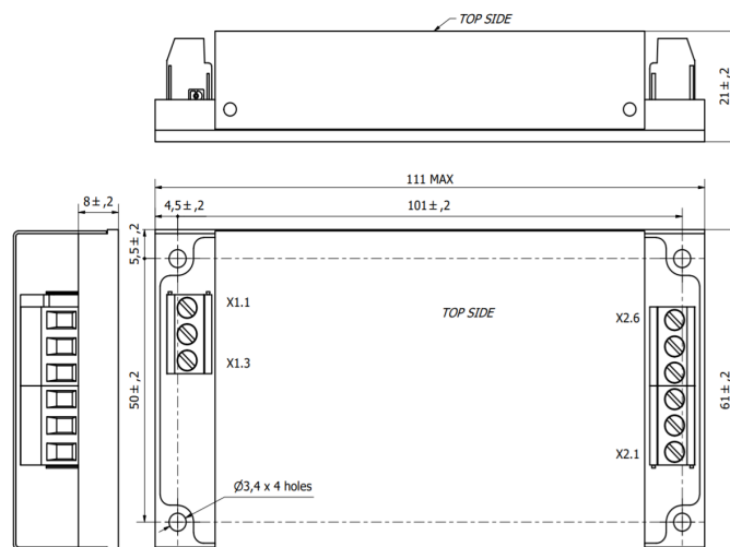
Рисунок Г.1 - Габаритные, присоединительные и установочные размеры модулей JETAs80, JETAs100, JETAs120, одноканальное исполнение (индекс S), с клеммными колодками (индекс C)
