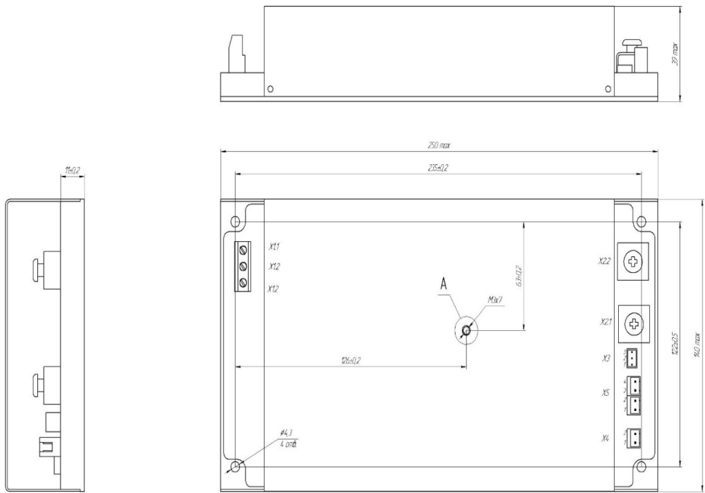
Рисунок И.1 - Габаритные, присоединительные и установочные размеры модулей JETAs1500, с клеммными колодками (индекс C)
