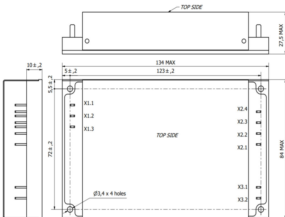
Рисунок Д.4 - Габаритные, присоединительные и установочные размеры модулей JETAs150, JETAs250, JETAs300, двухканальное исполнение (индекс D), с ножевыми контактами (индекс Н)
