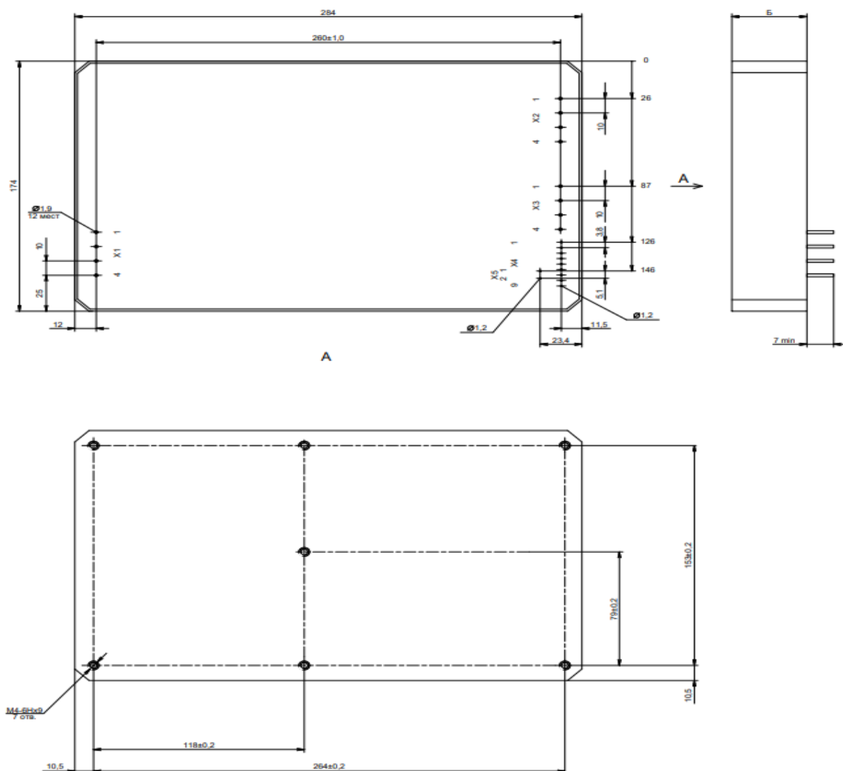
Рисунок К.2 - Габаритные, присоединительные и установочные размеры модуля JETAs2000, с ножевыми контактами (индекс Н)
