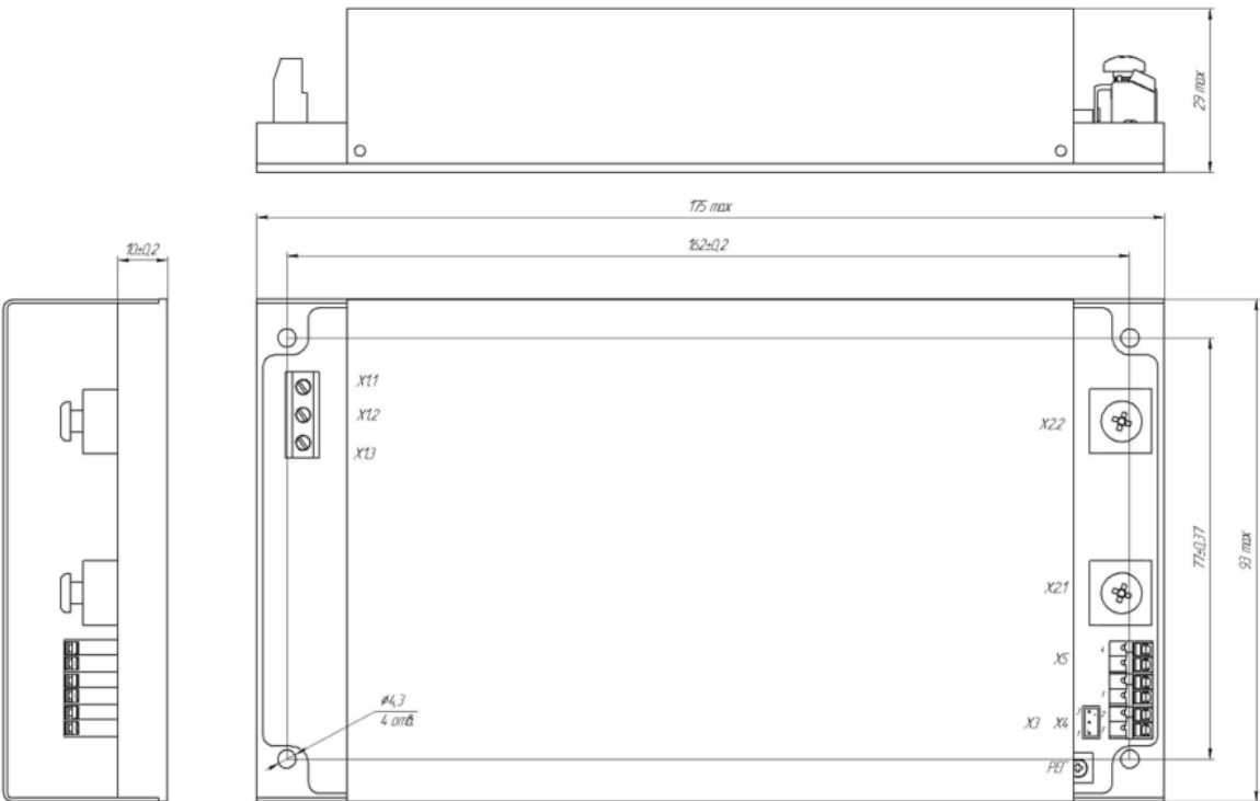
Рисунок Е.1 - Габаритные, присоединительные и установочные размеры модулей JETAs500, JETAs600, JETAs700, одноканальное исполнение (индекс S), с клеммными колодками (индекс C)
