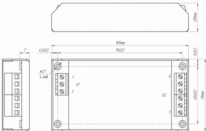
Рисунок В.3 - Габаритные, присоединительные и установочные размеры модулей JETAs30, JETAs40, JETAs60, трехканальное исполнение (индекс Т), с клеммными колодками (индекс С)
