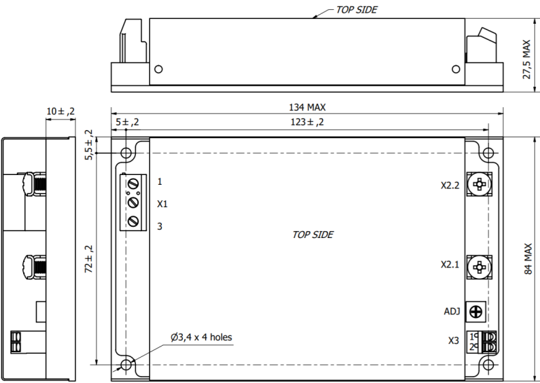
Рисунок Д.1 - Габаритные, присоединительные и установочные размеры модулей JETAs150, JETAs250, JETAs300, одноканальное исполнение (индекс S), с клеммными колодками (индекс C)
