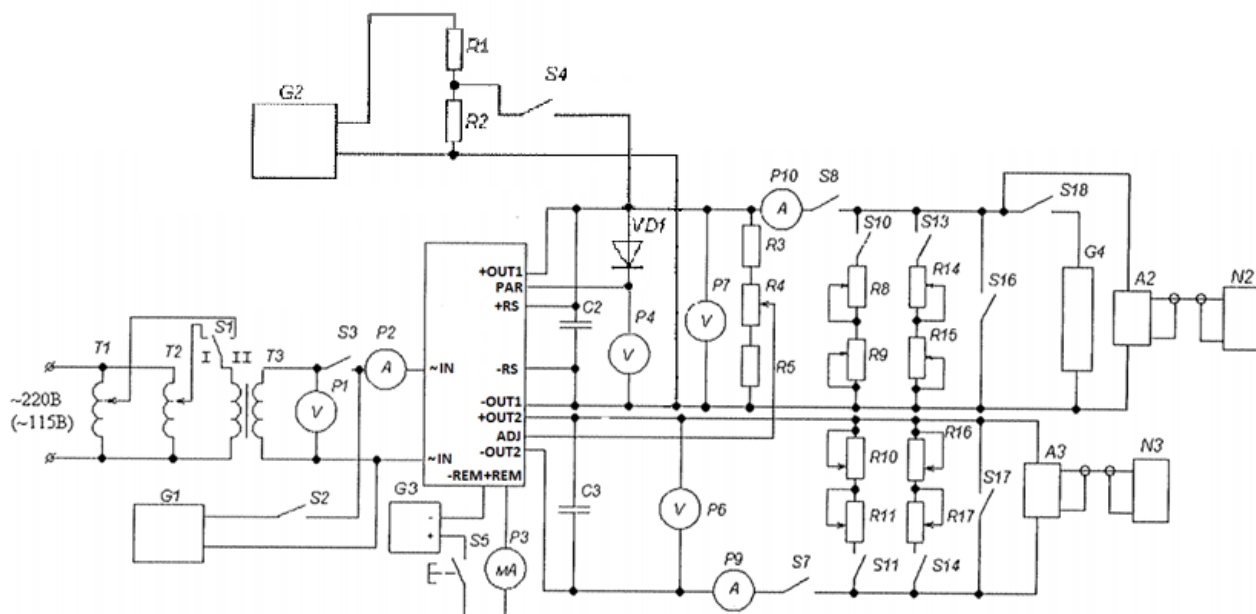
Рисунок А.1 – Схема измерений электрических параметров модулей
