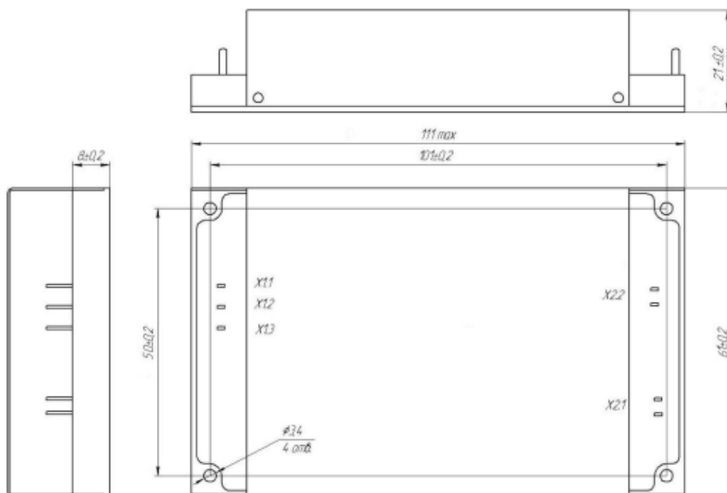
Рисунок Г.4 - Габаритные, присоединительные и установочные размеры модулей JETAs80, JETAs100, JETAs120, одноканальное исполнение (индекс S), с ножевыми контактами (индекс Н)
