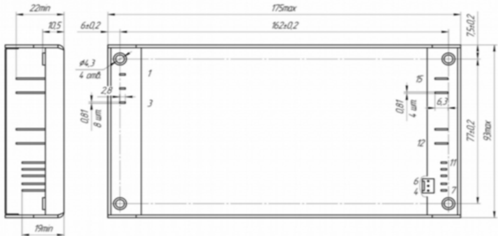
Рисунок Е.3 - Габаритные, присоединительные и установочные размеры модулей JETAs500, JETAs600, JETAs700, одноканальное исполнение (индекс S), с ножевыми контактами (индекс H)
