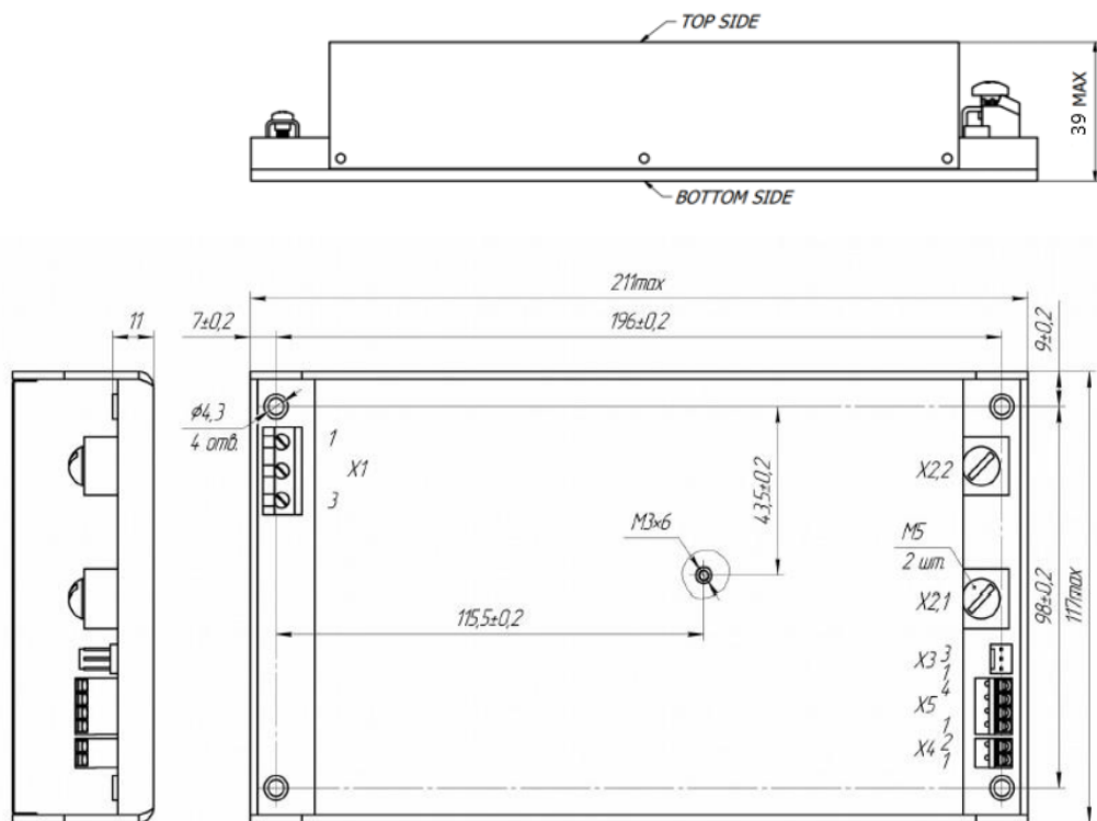
Рисунок Ж.1 - Габаритные, присоединительные и установочные размеры модулей JETAs1000, JETAs1200, с клеммными колодками (индекс С)
