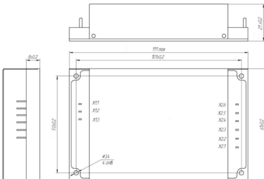
Рисунок Г.6 - Габаритные, присоединительные и установочные размеры модулей JETAs80, JETAs100, JETAs120, трехканальное исполнение (индекс Т), с ножевыми контактами (индекс Н)
