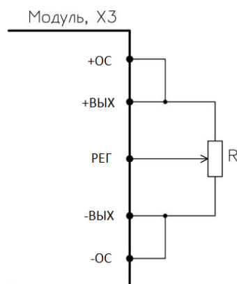
Рисунок 9.6 – Схема подключения внешнего потенциометра, для использования подстройки выходного напряжения с помощью вывода РЕГ
