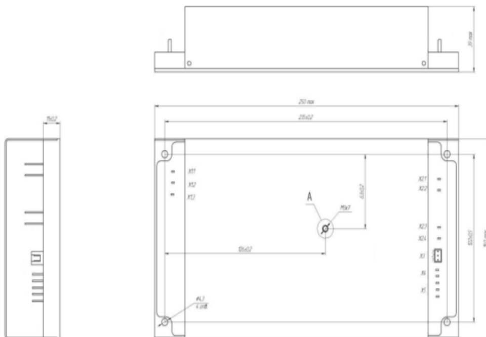
Рисунок И.2 - Габаритные, присоединительные и установочные размеры модуля JETAs1500, с ножевыми контактами (индекс Н)
