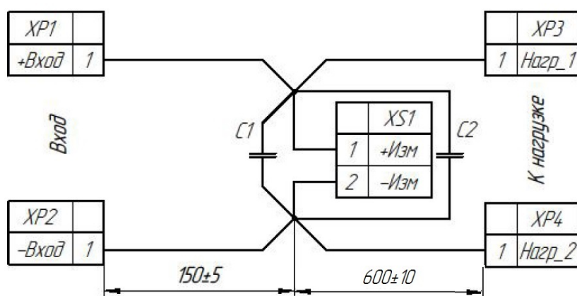
Рисунок 7.1 – Приспособление для измерения пульсаций выходного напряжения
