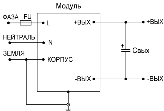
Рисунок 9.3 – Типовая схема включения одноканального модуля
