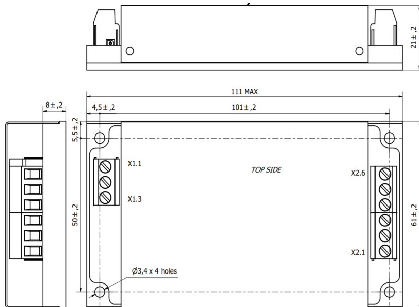
Рисунок Г.3 - Габаритные, присоединительные и установочные размеры модулей JETAs80, JETAs100, JETAs120, трехканальное исполнение (индекс Т), с клеммными колодками (индекс С)
