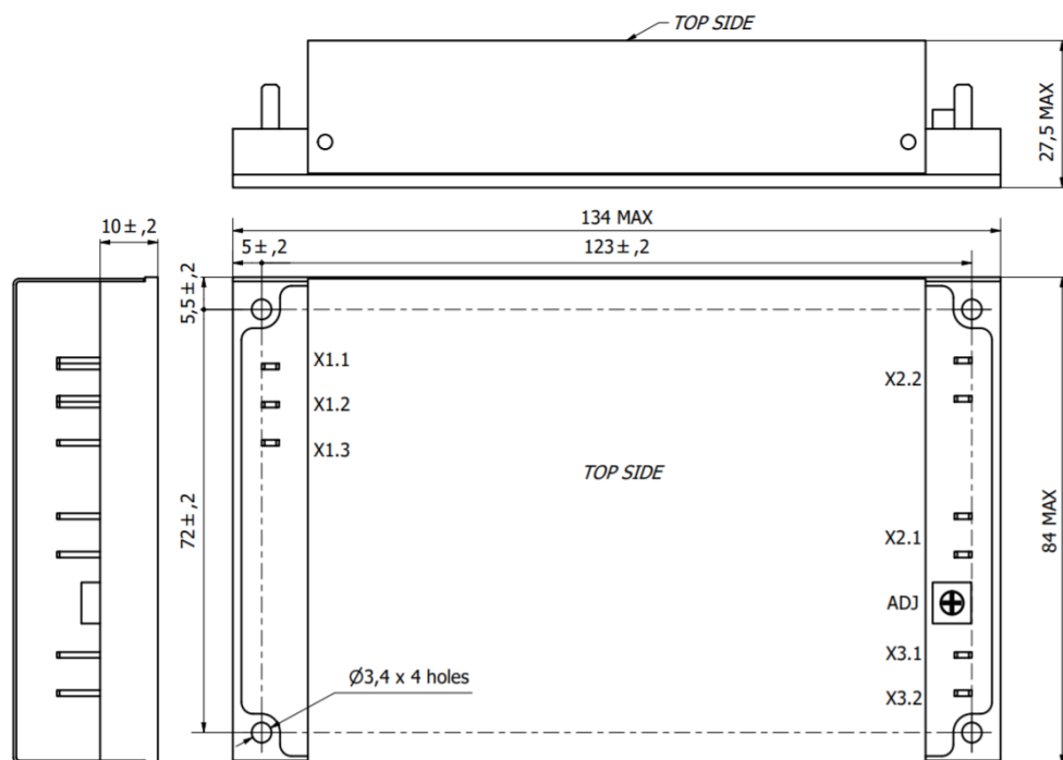
Рисунок Д.3 - Габаритные, присоединительные и установочные размеры модулей JETAs150, JETAs250, JETAs300, одноканальное исполнение (индекс S), с ножевыми контактами (индекс Н)
