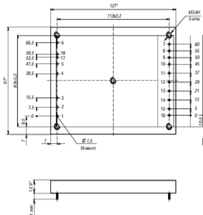
Корпус без фланцев
