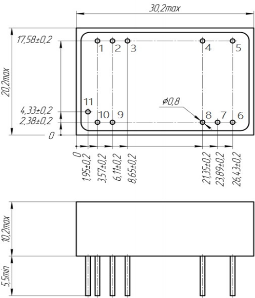
Рисунок В.2 - Габаритные, присоединительные и установочные размеры модуля TESDs15, одноканальное исполнение (индекс S), без фланцев (индекс C)
