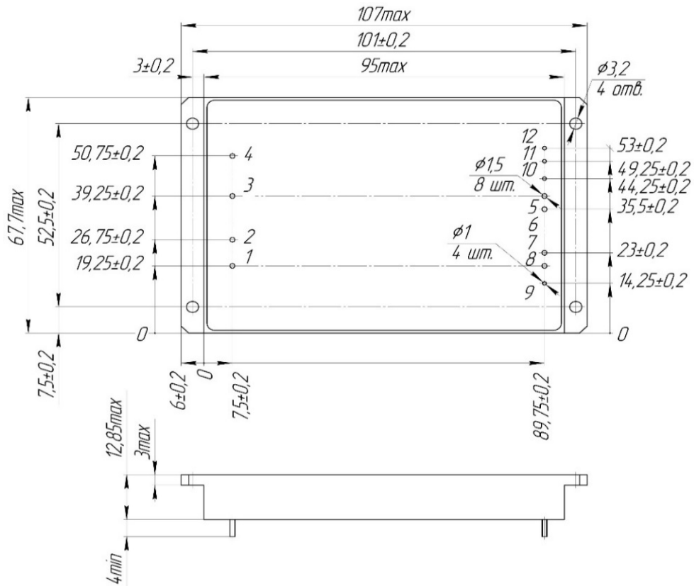
Рисунок И.1 - Габаритные, присоединительные и установочные размеры модуля TESDs500, одноканальное исполнение (индекс S), с фланцами (индекс U)
