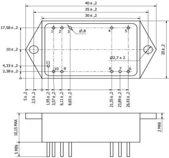
Рисунок В.1 - Габаритные, присоединительные и установочные размеры модуля TESDs15 одноканальное исполнение (индекс S), с фланцами (индекс U)
