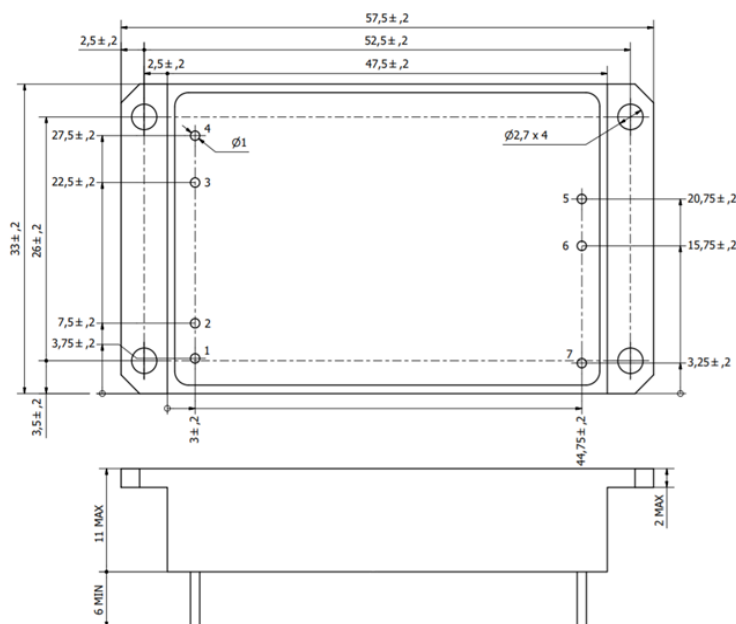
Рисунок Д.1 - Габаритные, присоединительные и установочные размеры модулей TESDs50, TESDs60, одноканальное исполнение (индекс S), с фланцами (индекс U)
