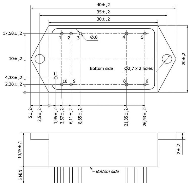
Рисунок В.3 - Габаритные, присоединительные и установочные размеры модуля TESDs15, двухканальное исполнение (индекс D), с фланцами (индекс U)
