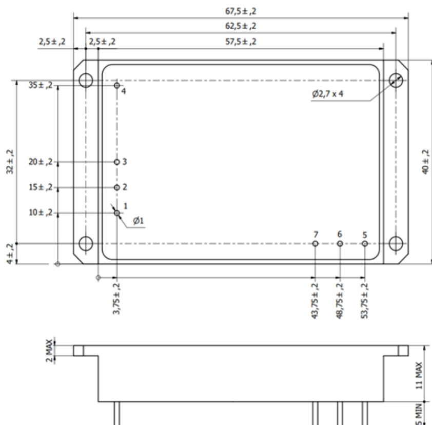
Рисунок Е.1 - Габаритные, присоединительные и установочные размеры модулей TESDs120, TESDs150, одноканальное исполнение (индекс S), с фланцами (индекс U)
