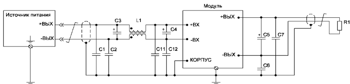
Рисунок 7.1 – Схема включения модуля без применения модуля фильтра
