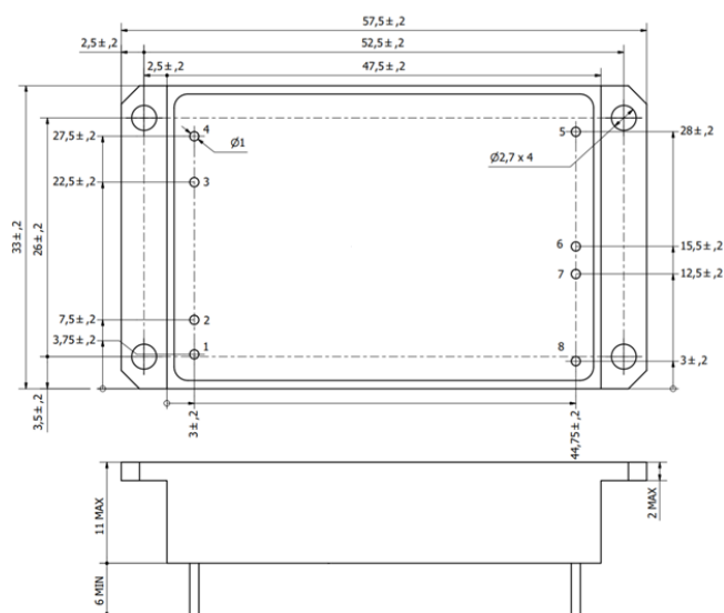
Рисунок Д.2 - Габаритные, присоединительные и установочные размеры модулей TESDs50, TESDs60, двухканальное исполнение (индекс D), с фланцами (индекс U)
