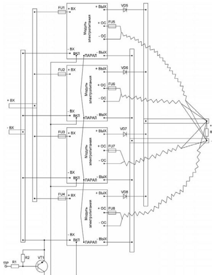
Рисунок 7.5 – Схема подключения модулей электропитания при параллельной работе
