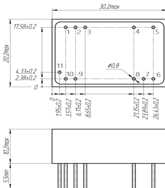
Рисунок В.4 - Габаритные, присоединительные и установочные размеры модуля TESDs15, двухканальное исполнение (индекс D), без фланцев (индекс C)
