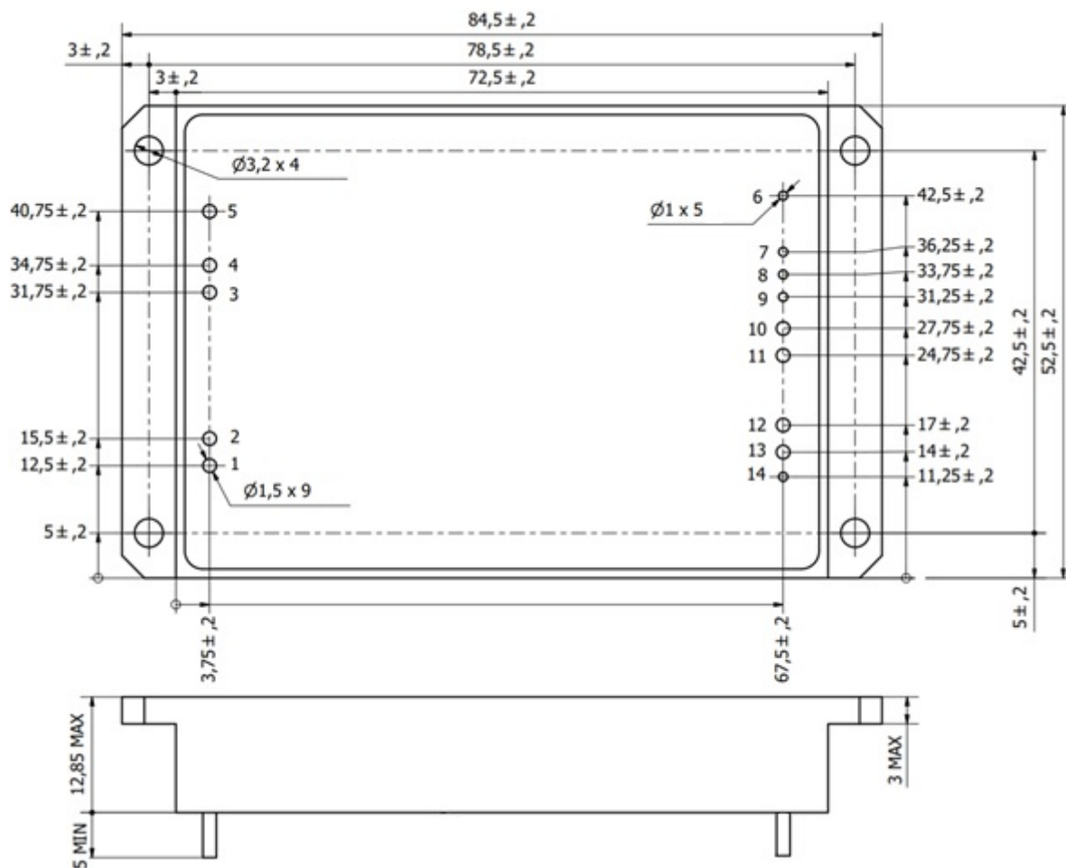
Рисунок Ж.1 - Габаритные, присоединительные и установочные размеры модулей TEDSd250, TEDSd300, одноканальное исполнение (индекс S), с фланцами (индекс U)
