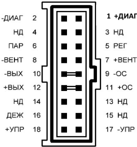
Рисунок Ж.2 – Ответная часть разъема X3
