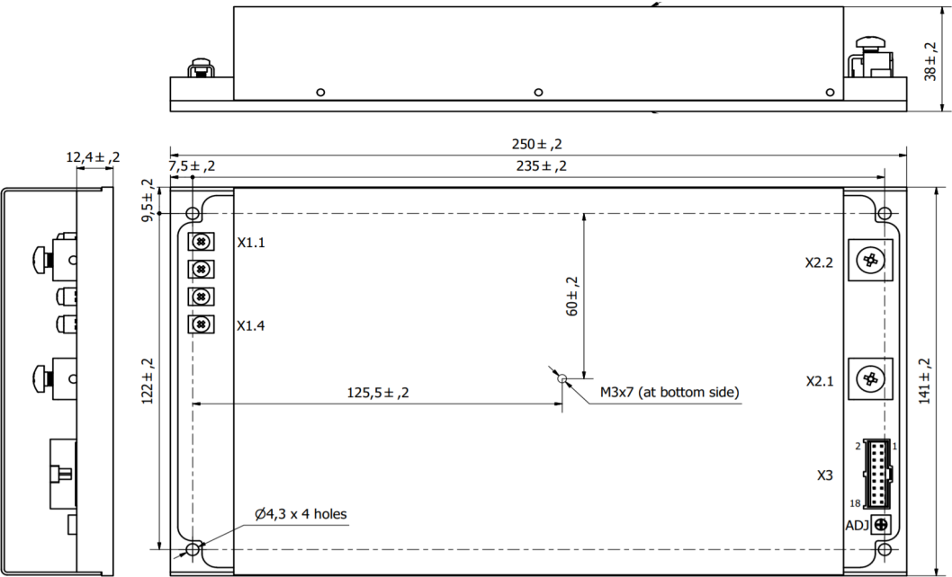
Рисунок Д.1 - Габаритные, присоединительные и установочные размеры модуля ТПС3000, одноканальное исполнение (индекс С), с клеммными колодками (индекс К)
