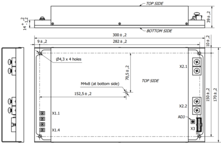
Рисунок Ж.1 - Габаритные, присоединительные и установочные размеры модуля ТПС5000, одноканальное исполнение (индекс С), с клеммными колодками (индекс К)
