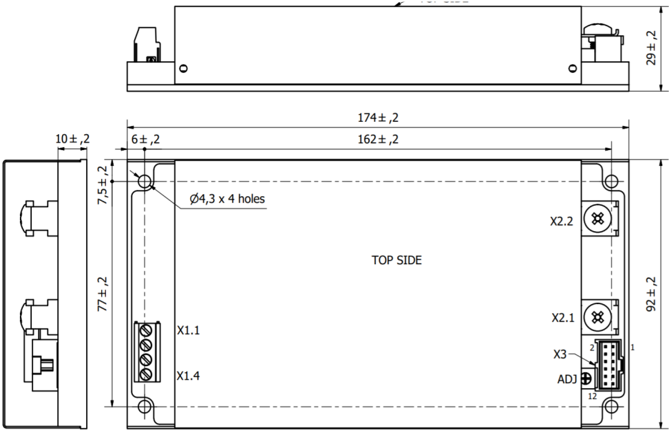
Рисунок В.1 - Габаритные, присоединительные и установочные размеры модуля ТПС1000, одноканальное исполнение (индекс С), с клеммными колодками (индекс К)
