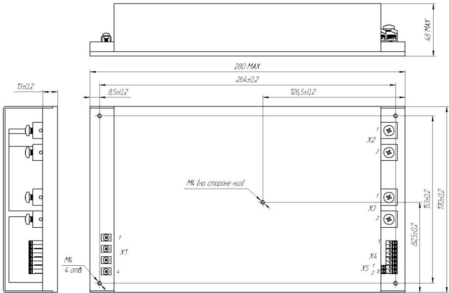
Рисунок Е.1 - Габаритные, присоединительные и установочные размеры модуля ТПС4000, одноканальное исполнение (индекс С), с клеммными колодками (индекс К)
