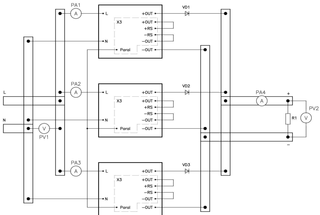
Рисунок 9.8 – Резервированная система, построенная по принципу N+M с равнозначными модулями
