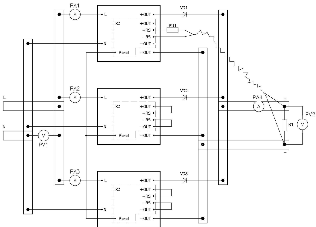
Рисунок 9.10 – Система, построенная по принципу «ведущий-ведомый»
