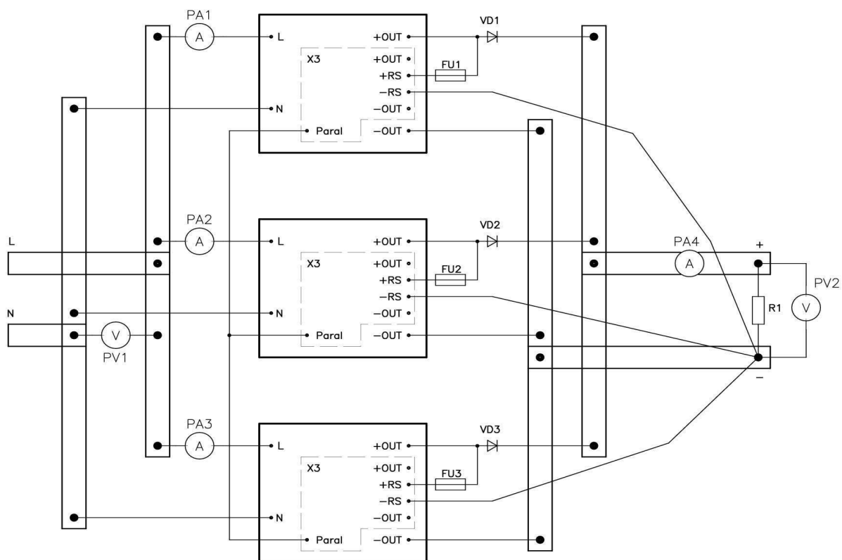
Рисунок 9.9 – Резервированная система, построенная по принципу N+M с равнозначными модулями и использованием выносной обратной связи
