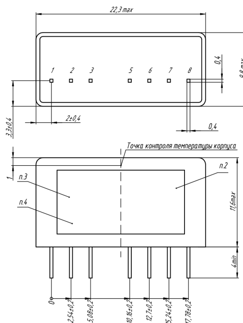
Габаритный чертёж ТЕНс3.
