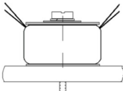
Рисунок А.1 (Крепление винтом)
