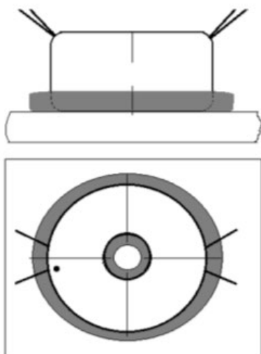
Рисунок А.3 (Крепление подклейкой)
