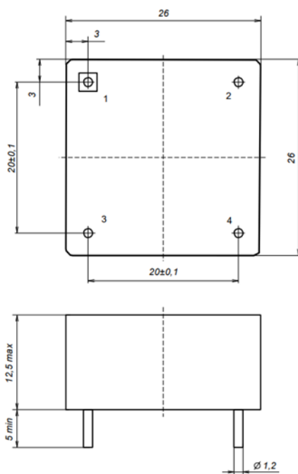
Рисунок В.4 – Габаритные размер дросселей ДФТК120-2М(Н)/х, ДФТК240-2М(Н)/х
