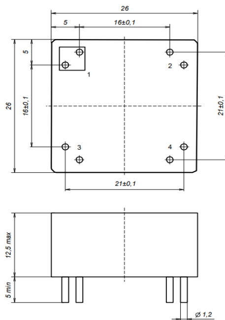
Рисунок В.5 – Габаритные размеры дросселей ДФТК60-2А(В, Д, Р)/х, ДФТК120-2А(В, Д, Р)/х, ДФТК240-2В(Д), ДФТПК60-2/х
