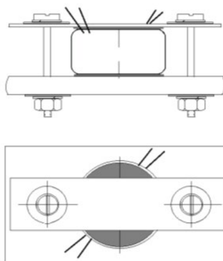
Рисунок А.4 (Крепление пластиной)
