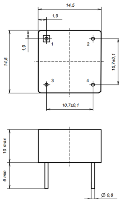
Рисунок В.1 – Габаритные размер дросселей ДФТК7,5-2х/х, ДФТПК7,5-2/х
