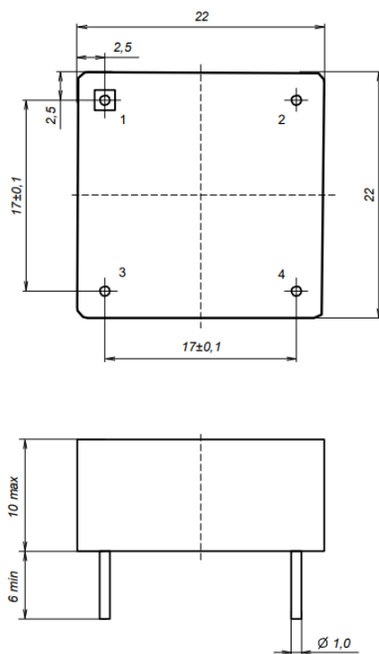
Рисунок В.3 – Габаритные размер дросселей ДФТК30-2х/х, ДФТК60-2М(Н)/х, ДФТПК30-2/х
