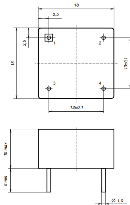
Рисунок В.2 – Габаритные размер дросселей ДФТК15-2х/х, ДФТПК15-2/х
