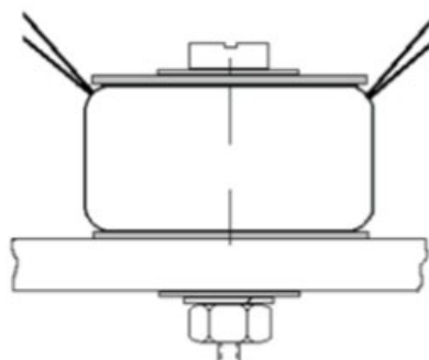
Рисунок А.2 (Крепление винтом и гайкой)
