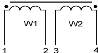
Рисунок 3.2 – Схема дросселей серии ДФТП, ДФТПК, выполненных по двухобмоточной схеме
