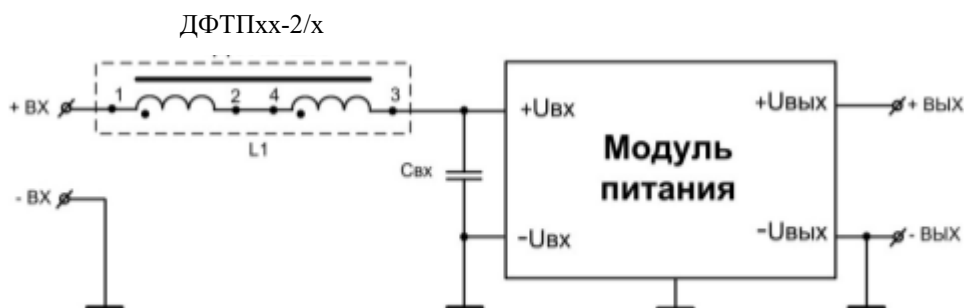
Рисунок 7.3 – Установка дросселей с модулем питания в однопроводную сеть
