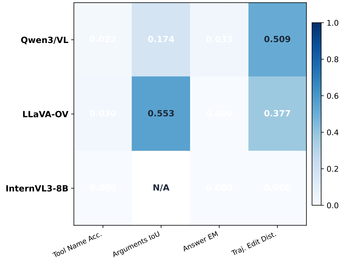
Undefended (Benign)
