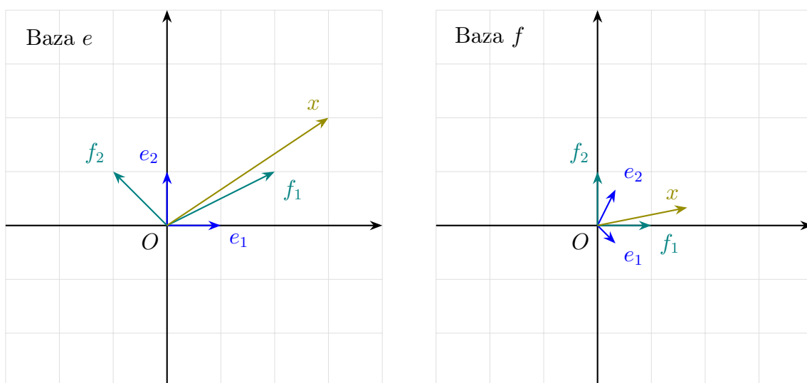
Slika 9.6: Promena baze
