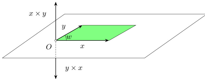
Slika 9.2: Vektorski proizvod
