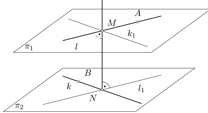
Slika 10.1: Zajednička normala mimoilaznih pravih
