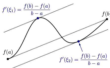
Slika 11.2: Lagranžova teorema
