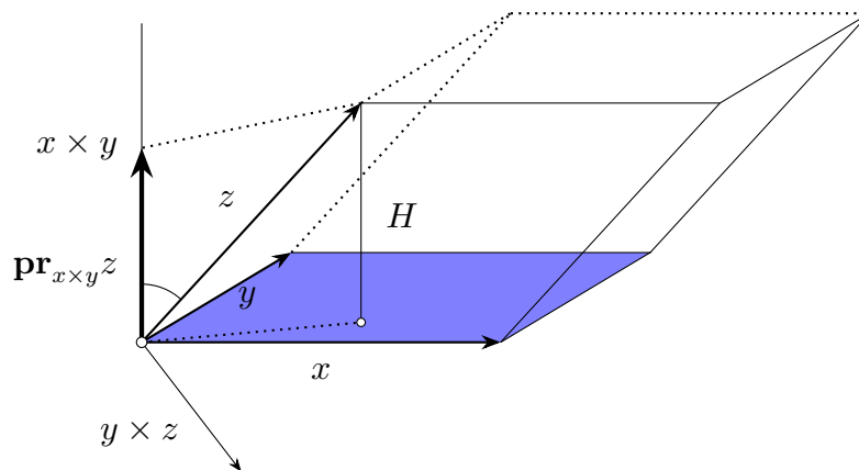
Slika 9.3: Mešoviti proizvod
