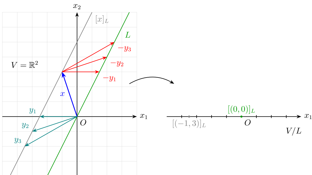
Slika 9.5: Faktor prostor
