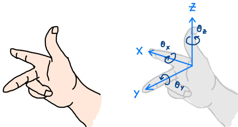
Slika 9.1: Pravilo desne ruke
