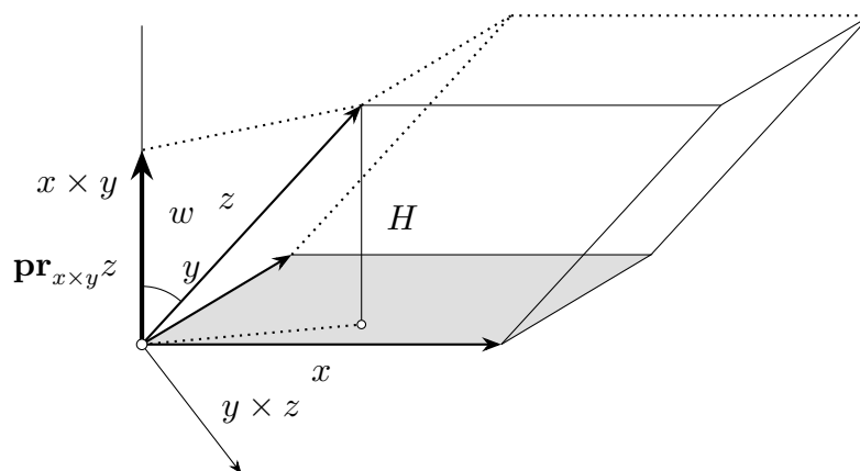
Slika 9.4: Mešoviti proizvod
