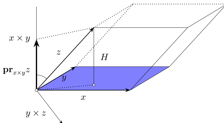
Slika 9.3: Mešoviti proizvod
