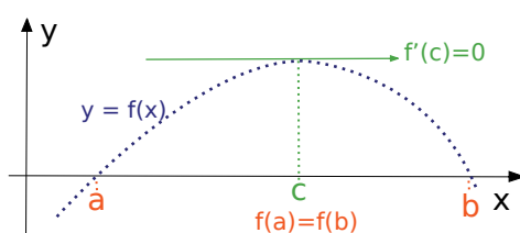
Slika 10.1: Rolova teorema
