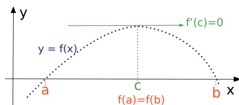
Slika 14.1: Rolova teorema
