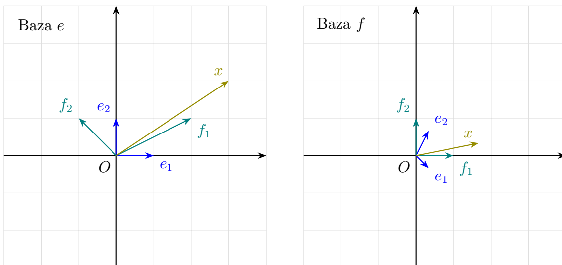
Slika 11.6: Promena baze
