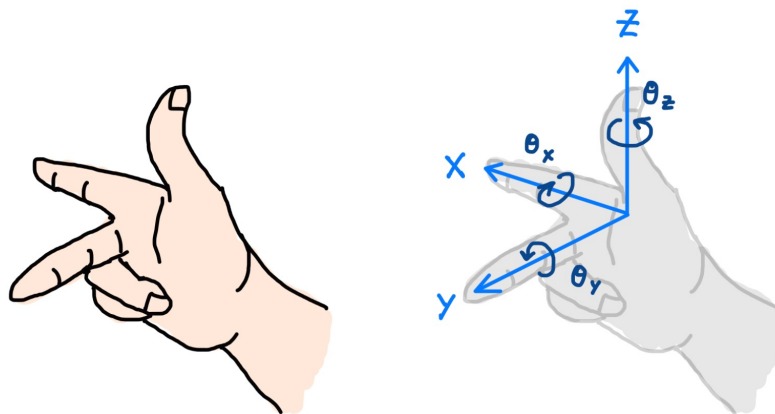
Slika 11.1: Pravilo desne ruke
