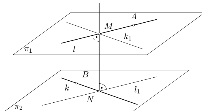
Slika 12.1: Zajednička normala mimoilaznih pravih
