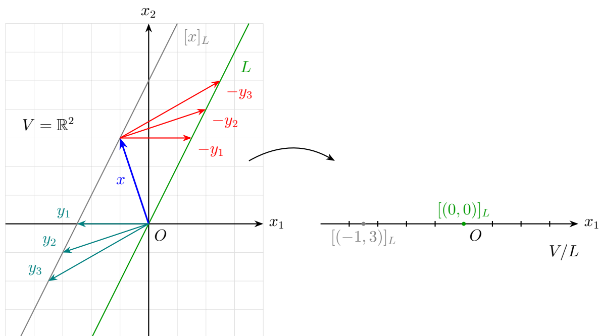
Slika 11.5: Faktor prostor
