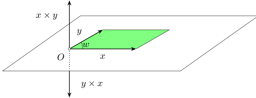
Slika 11.2: Vektorski proizvod
