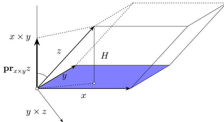
Slika 11.3: Mešoviti proizvod
