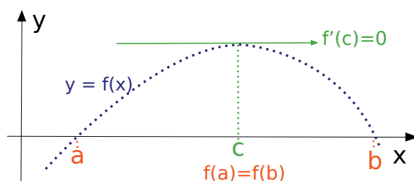
Slika 9.1: Rolova teorema
