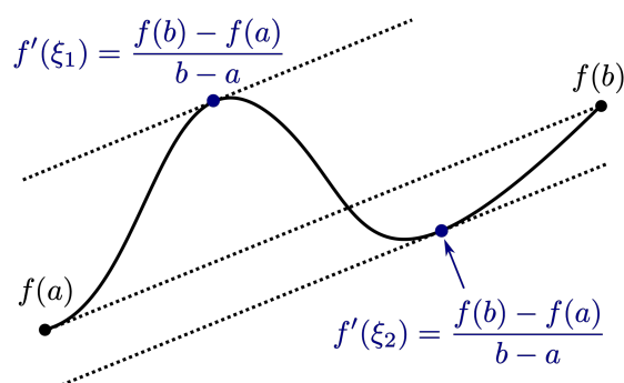
Slika 9.2: Lagranžova teorema
