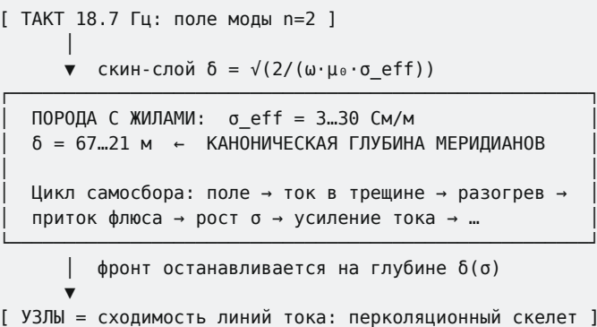
Рис. 3.1 — Самосбор меридианной сети: скин-слой как равновесный фронт
