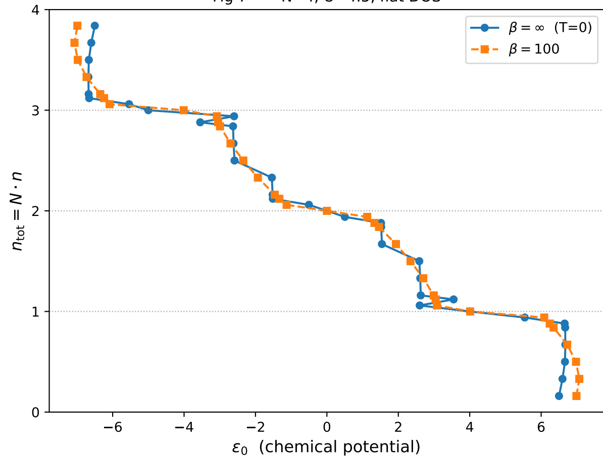
Fig 7 — N=4 , U=4.5 , flat DOS
