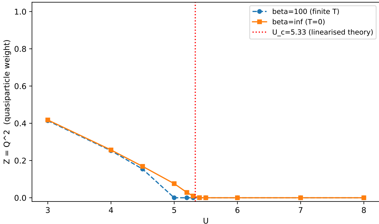
MIT scan \alpha=1 n=0.333 flat DOS ( W=1 )
