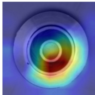
MobileNetV2
