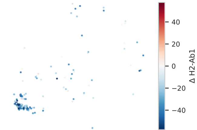
C Predicted \Delta H2-Ab1 (in-silico KO)
