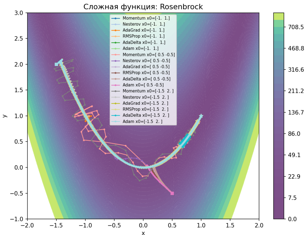
Рис. 8: Траектории на функции Розенброка (3 стартовые точки: (-1, 1) , (0.5, -0.5) , (-1.5, 2) ).
