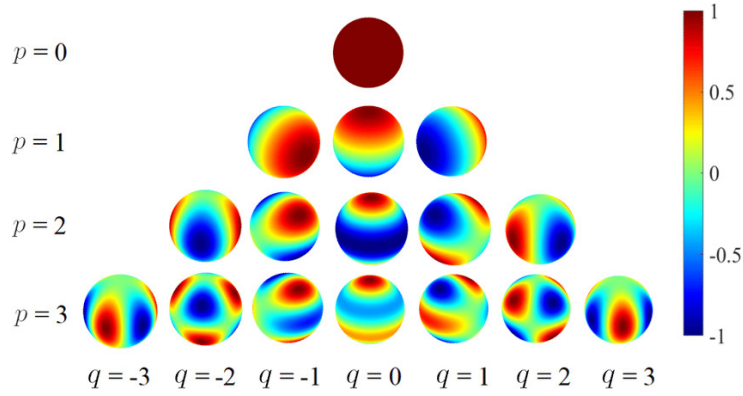
Slika 3: Realni sferični harmonici Y_p^q na sferi, za stepene p = 0 do 3 (vrste) i redove q = -p, \dots, p (kolone); boja označava vrednost funkcije (plavo -1 , crveno +1 ). Stepen p = 0 (vrh) je konstanta i jedini se koristi u ovom radu, dok viši stepeni uvode sve finije ugaone varijacije [6].
