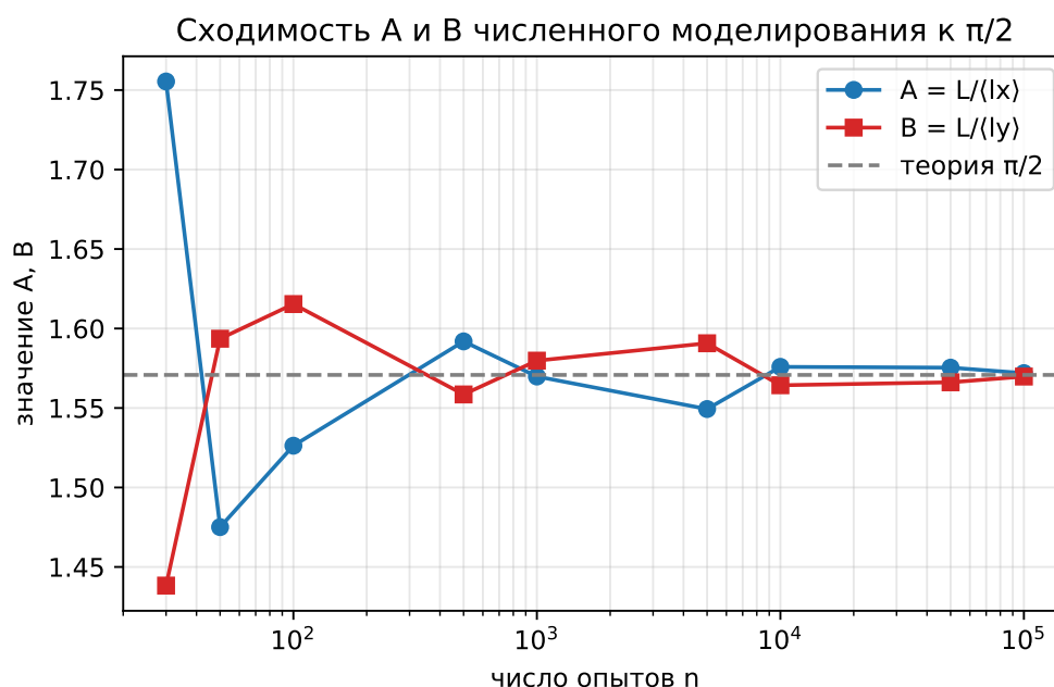
Рис. 2 — Сходимость значений A и B , полученных путем численного моделирования, к теоретическому значению \pi/2 при увеличении числа опытов n (логарифмическая шкала по оси n ).
