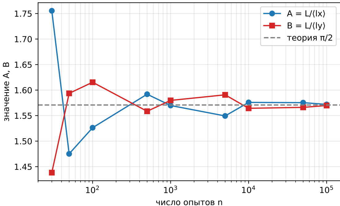
Сходимость A и B численного моделирования к \pi/2
