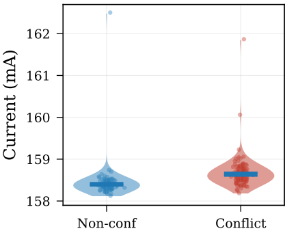
(d) VCCO_PSDDR Per-pair means
