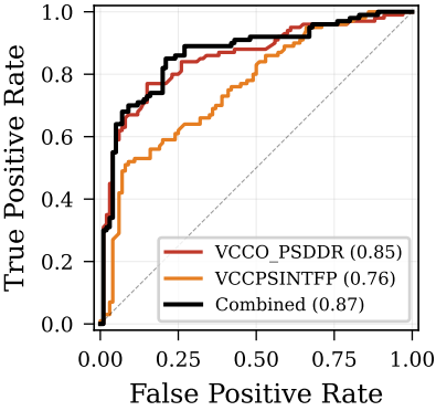
(f) ROC — Per-pair
