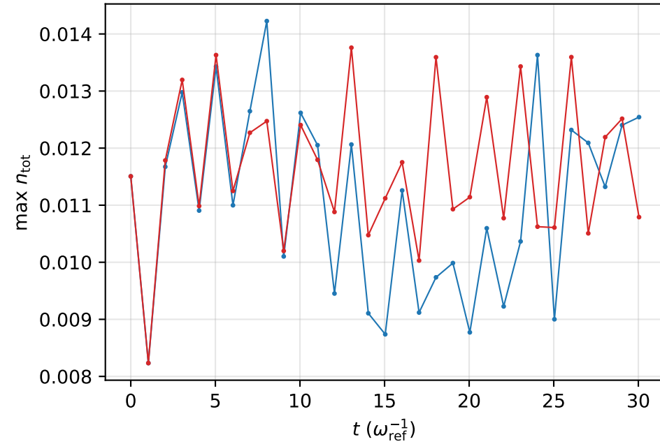
(d) peak density
