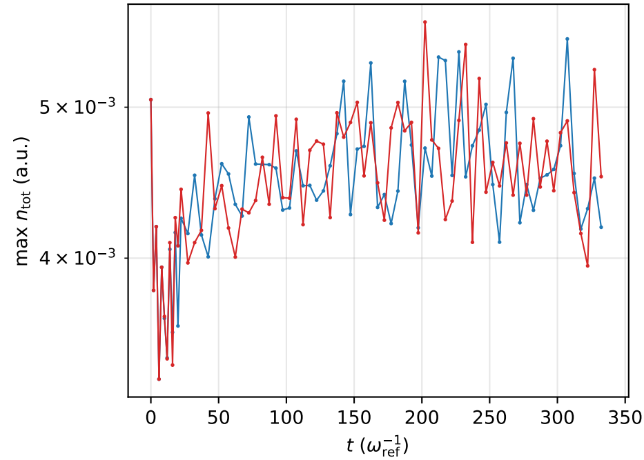
(d) peak density (sampled)
