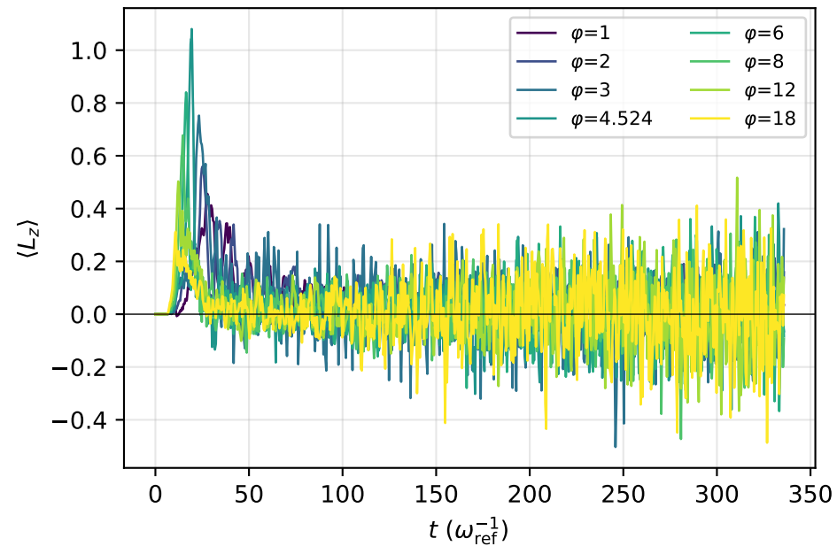
(a) orbital angular momentum (Berry connection)
