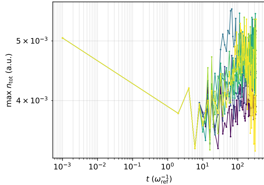
(d) peak density (sampled)
