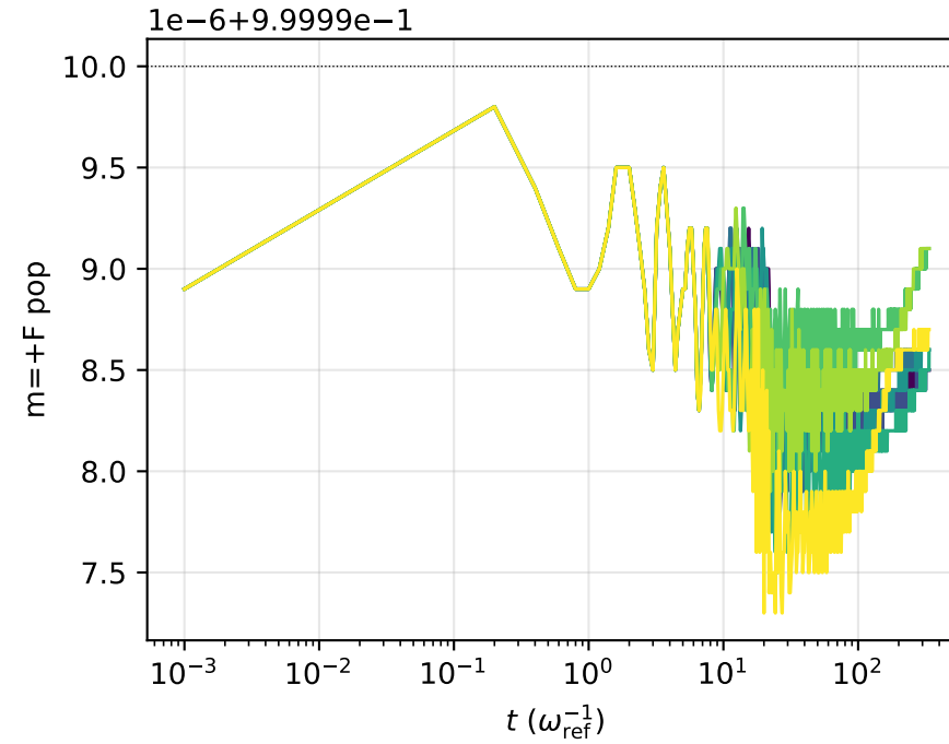
(e) m=+F population (Klaus freeze)
