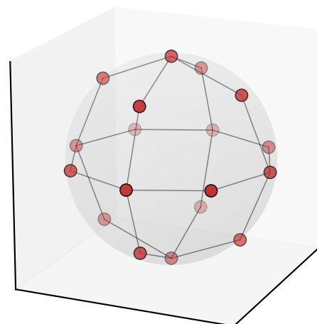
F=9 octa O:A 1 (supp) — 18 stars
