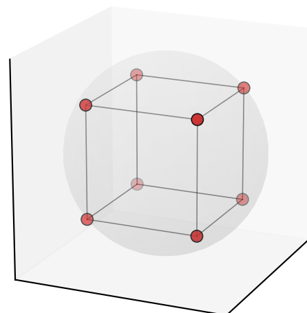
F=9 octa O:A 1 (supp) — 18 stars
