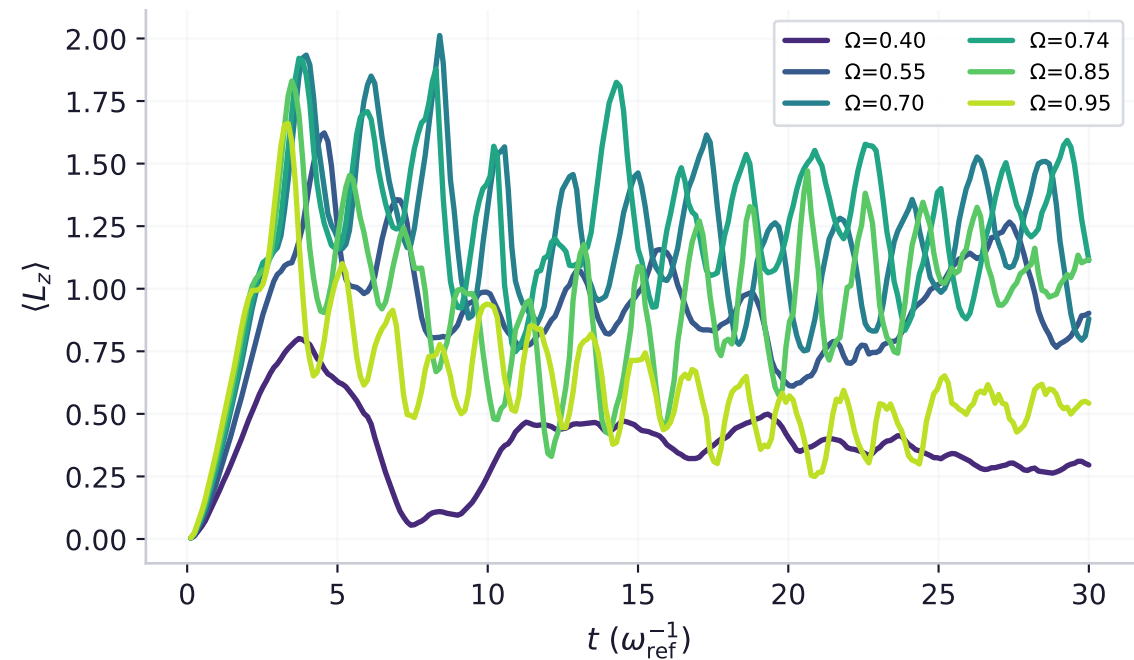
(d) threshold \Omega_c : circulation + vortices turn on
