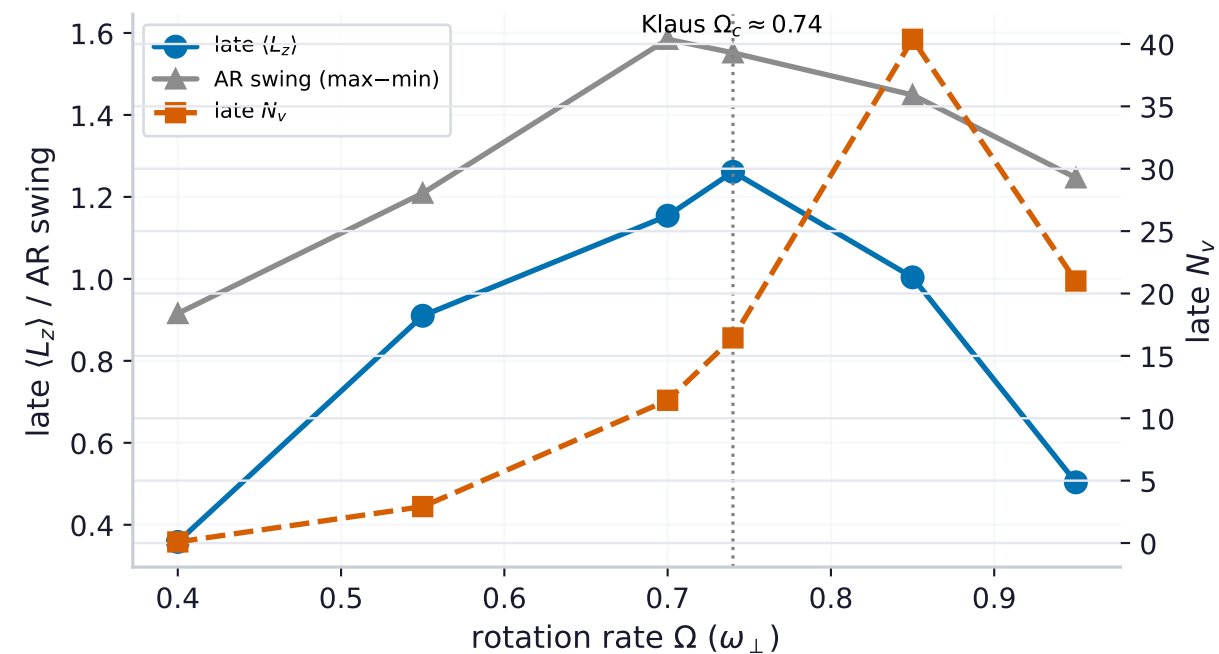
(d) threshold \Omega_c : circulation + vortices turn on
