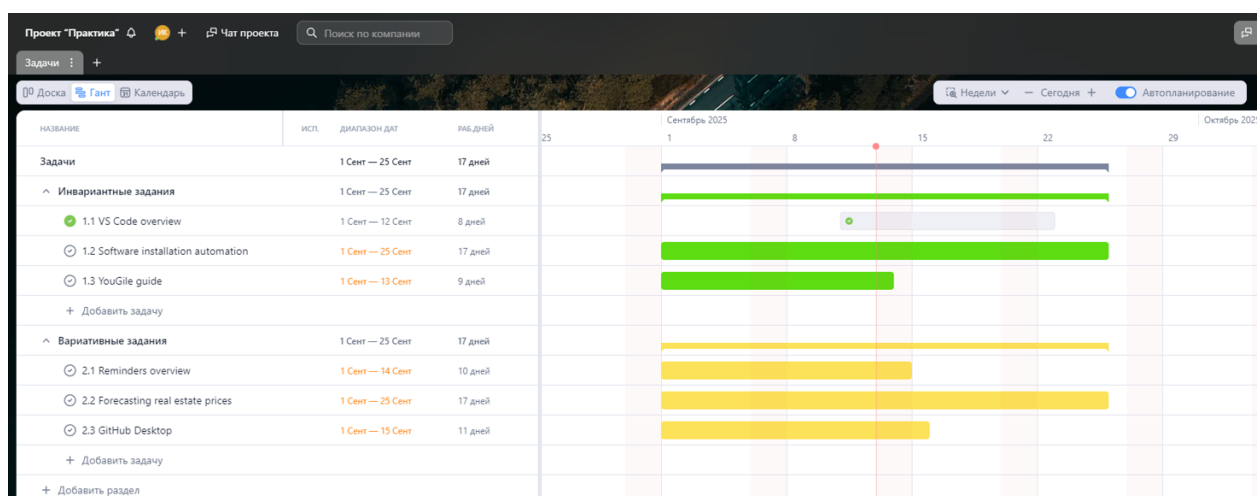
Рисунок 6 – Диаграмма Ганта
